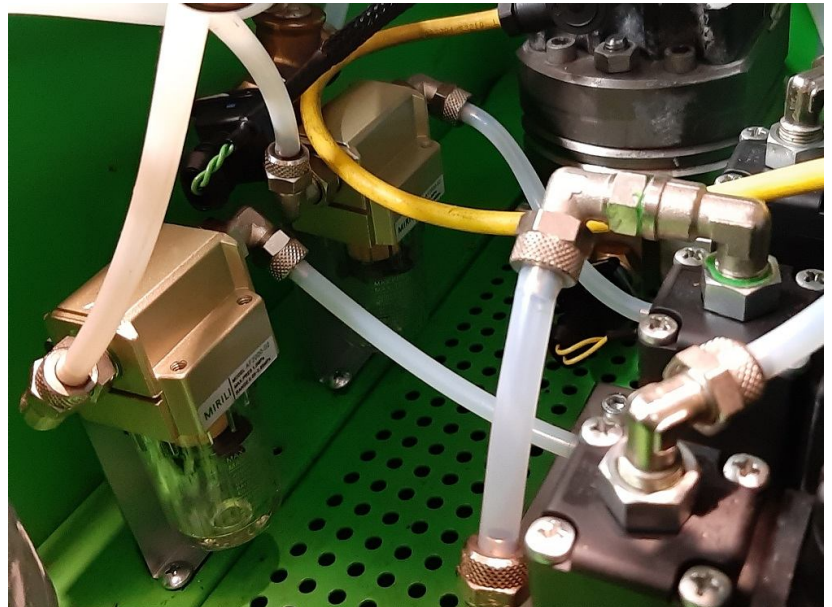
Esempio di installazione su Banco prova tipo 555-DDP
