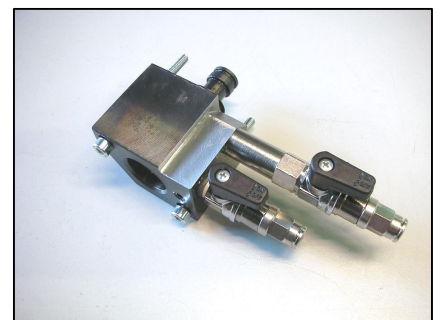
Adattatore pressione di tra- sferta regolata e non regolata con connessione universale da IMV COD.: 555-30-D
